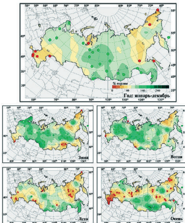
Рисунок 3.6 – Аномалии осадков на территории Российской Федерации в 2020 г., с указанием локализации 5%-х экстремумов (красные кружки) и 95%-х (зеленые кружки)
