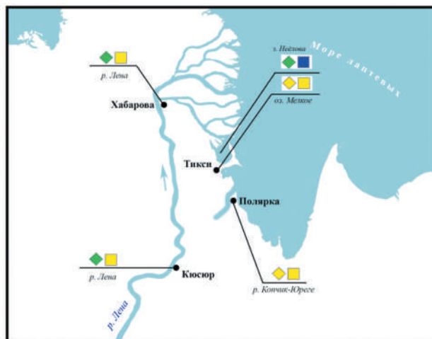
Рисунок 12.28 – Картограмма качества вод Республики Саха (Якутия) по гидробиологическим показателям в 2020 г.
