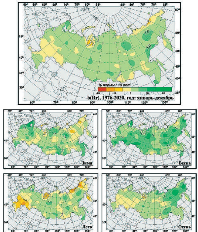
Рисунок 3.9 – Пространственные распределения локальных коэффициентов линейного тренда годовых и сезонных сумм атмосферных осадков за 1976–2020 гг. на территории Российской Федерации (%/10 лет)
