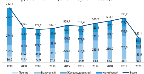
Рисунок 10.29 — Динамика пассажинооборота (без легкового такси) по видам транспорта общего пользования, 1990–2020 гг., млрд пассажиро-км
