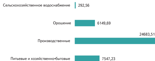
Рисунок 4.48 – Использование свежей воды для различных нужд в 2020 г., млн м 3 Источник: данные Росводресурсов
