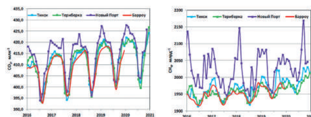
Рисунок 3.15 – Временной ход концентрации \text{CO}_2 и \text{CH}_4 на российских арктических станциях в сравнении с данными станции Барроу (Национальное управление по исследованию океанов и атмосферы Министерства торговли Соединенных Штатов Америки)
